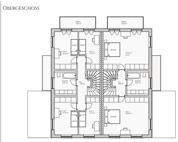
Grundriss Obergeschoss
