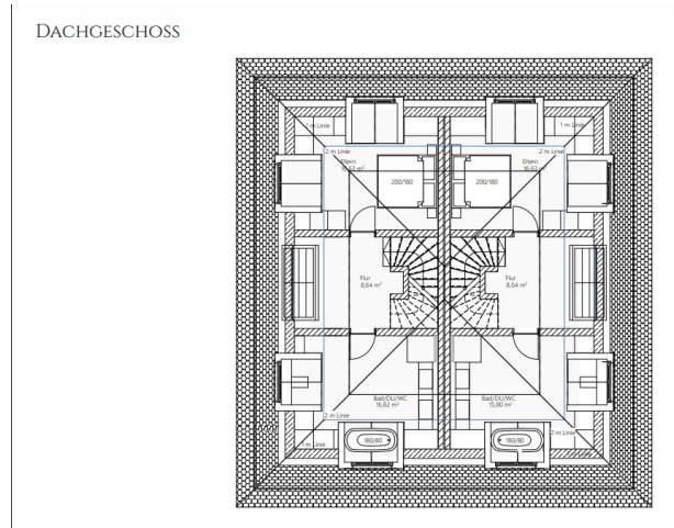
Grundriss Dachgeschoss
