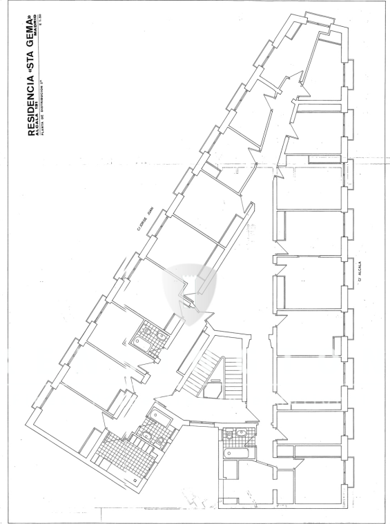
2ª planta
